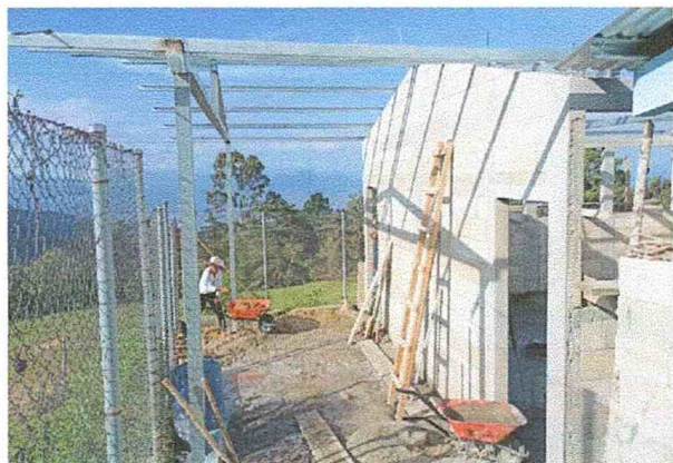
Foto 3: Colocación de costaneras del entechado de la estructura.
